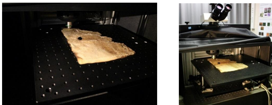
Figure 2 : Photographie du microscope d'optique non-linéaire du Laboratoire d'optique et biosciences (CNRS, École polytechnique – Institut Polytechnique de Paris, Inserm) avec un parchemin historique de la médiathèque de Chartres en cours d'analyse. (Crédit : M. Schmeltz, LOB).
