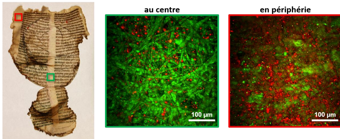
Figure 1 : Photographie d'un manuscrit sur parchemin issu du fonds de la bibliothèque de Chartres (Crédit : CNRS-IRHT). Images en fausses couleurs de microscopie optique non-linéaire avec les signaux de génération de seconde harmonique correspondant au collagène fibrillaire (en vert) et la fluorescence excitée à deux photons, liée à la dégradation du collagène (en rouge). Le centre du parchemin est bien conservé alors que la périphérie est davantage altérée.
